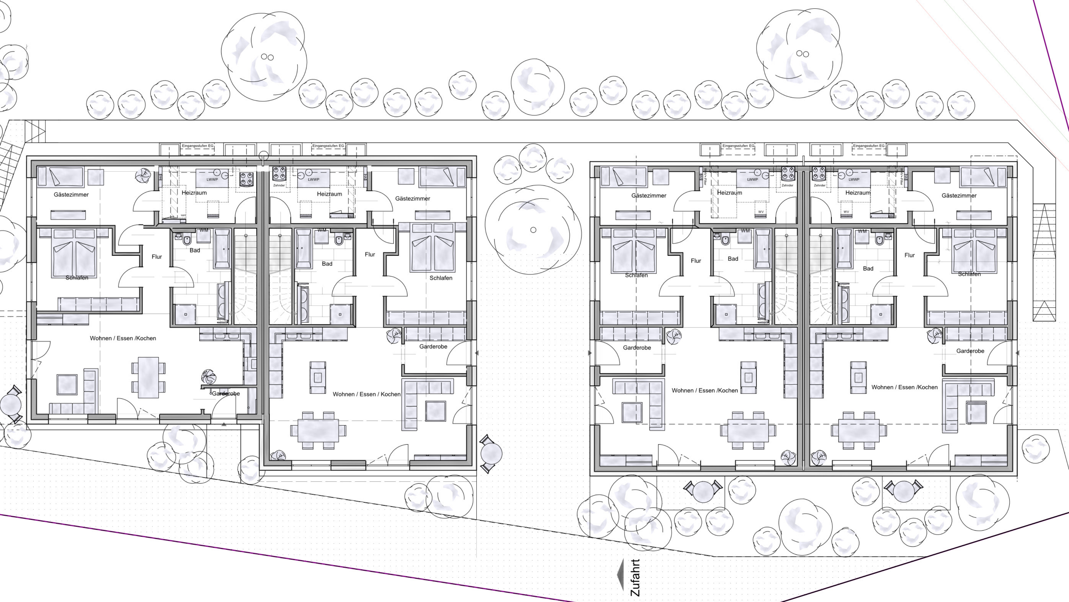
Doppelhaus 2
