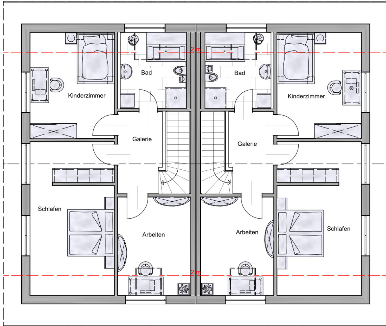
Balkon EG
